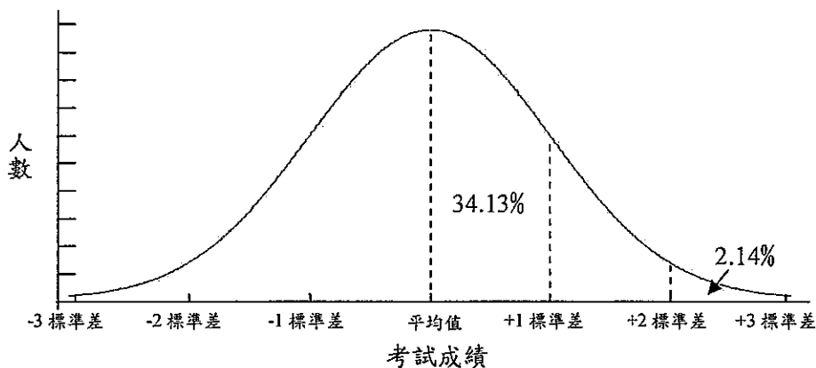
常態分配圖
