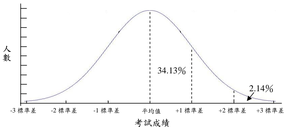
常態分配圖
